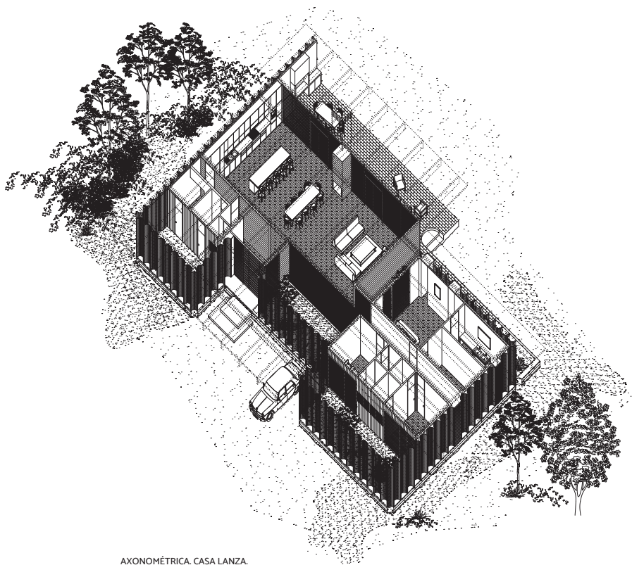
AXONOMÉTRICA. CASA LANZA.
