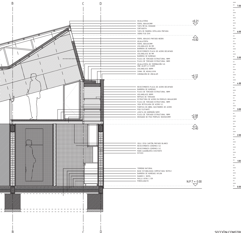
SECCIÓN CONSTRUCTIVA. CASA LAUTARO.
