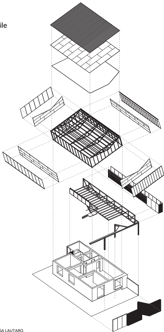
AXONOMÉTRICA. CASA LAUTARO.
